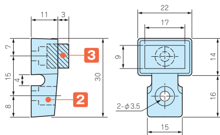
取付穴寸法図
